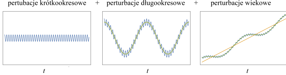
Rysunek 3.1: Typy perturbacji w zagadnieniach grawitacyjnych. Perturbacje krótkookresowe mogą wystąpić we wszystkich zmiennych, długookresowe we wszystkich oprócz L , wiekowe tylko w kątach l , g , h .
